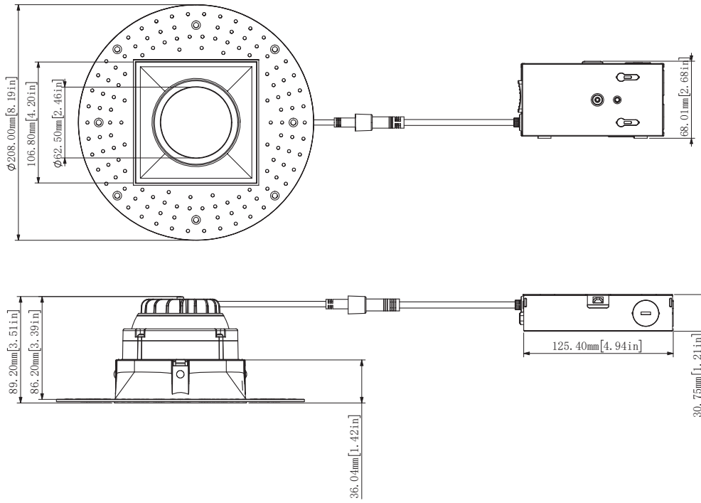
Technical Drawing: 8.19" (D) x 3.51" (W)
