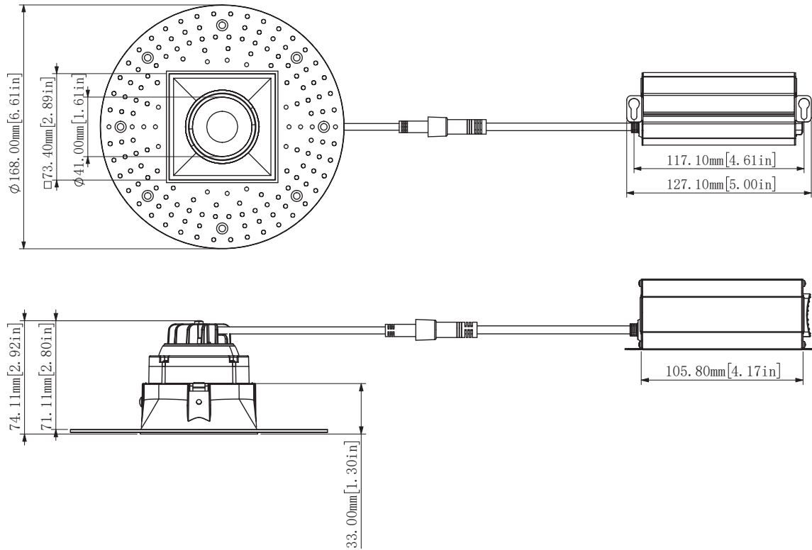
Technical Drawing: 6.61" (D) x 2.92" (W)
