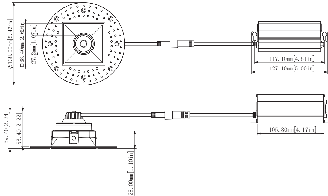
Technical Drawing: 5.43" (D) x 2.34" (W)
