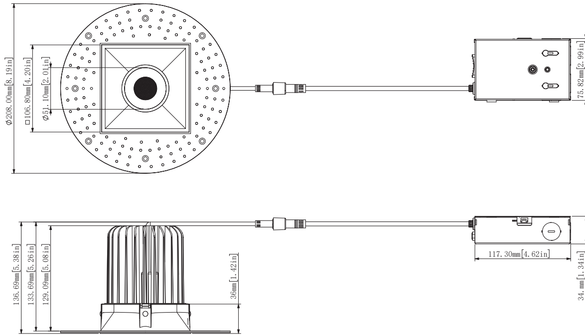
Technical Drawing: 8.19" (D) x 5.38" (W)
