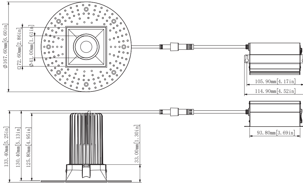
Technical Drawing: 6.6" (D) x 5.25" (W)
