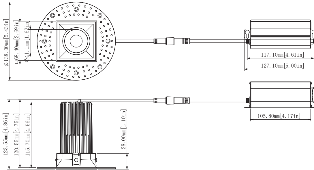
Technical Drawing: 5.43" (D) x 4.86" (W)
