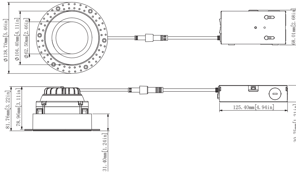
Technical Drawing: 5.46" (D) x 3.22" (W)
