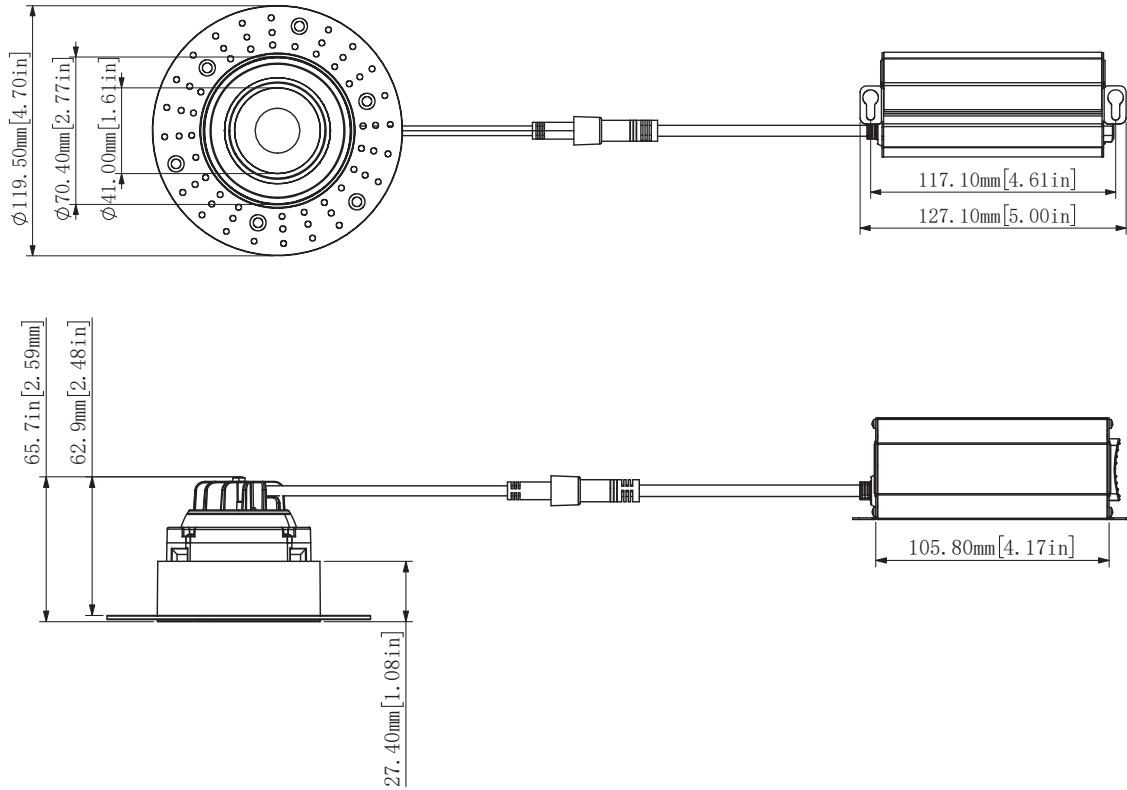
Technical Drawing: 4.7" (D) x 2.59" (W)
