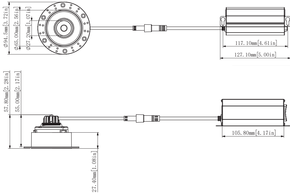
Technical Drawing: 3.72" (D) x 2.28" (W)
