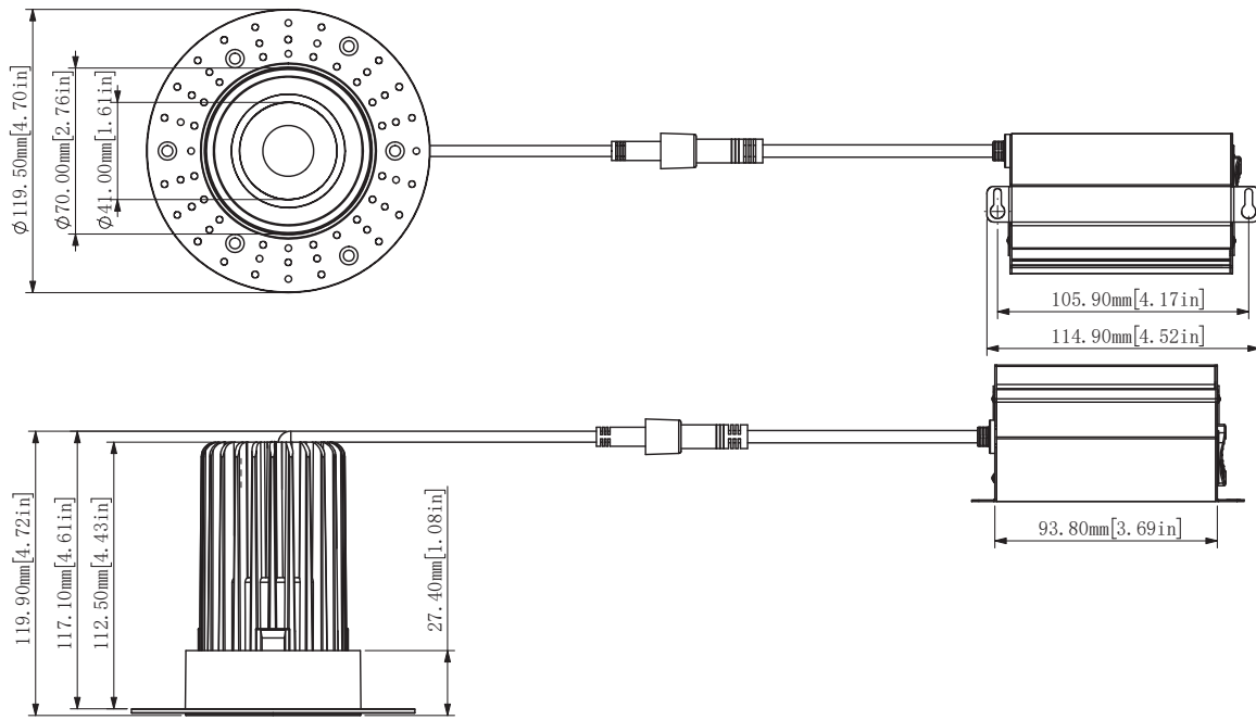
Technical Drawing: 4.7" (D) x 4.72" (W)
