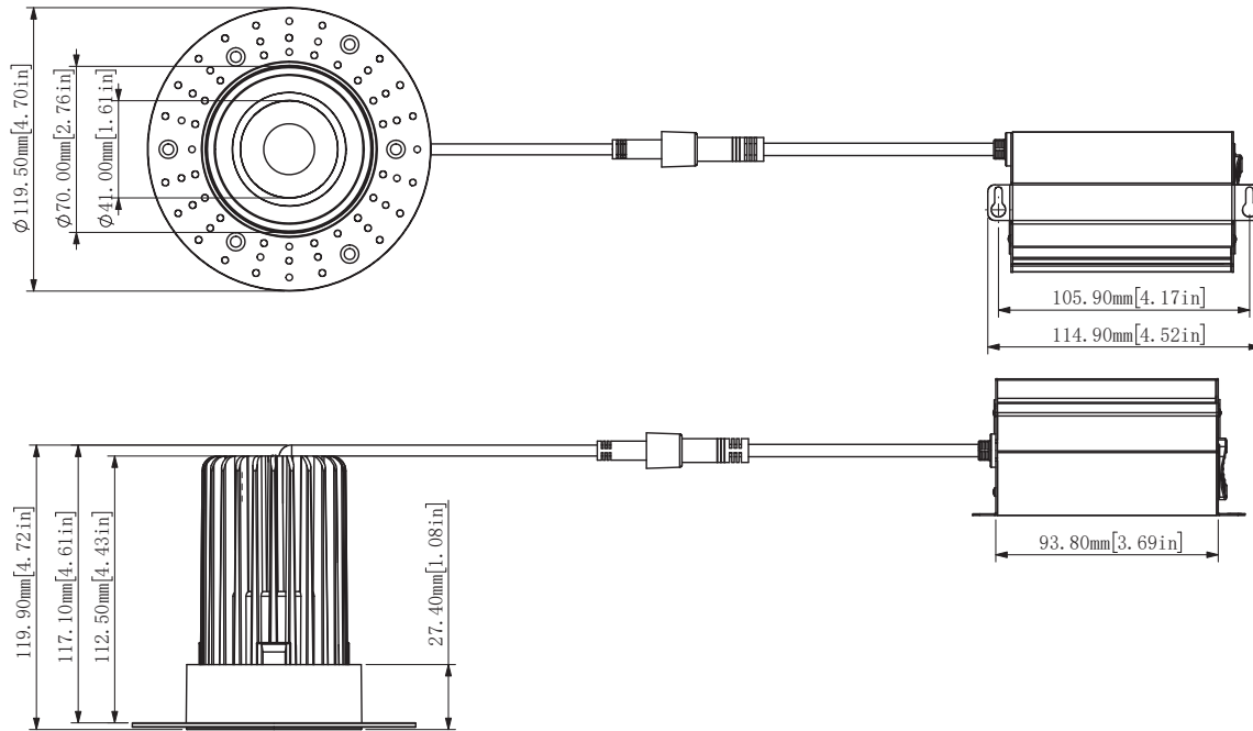
Technical Drawing: 4.7" (D) x 4.72" (W)
