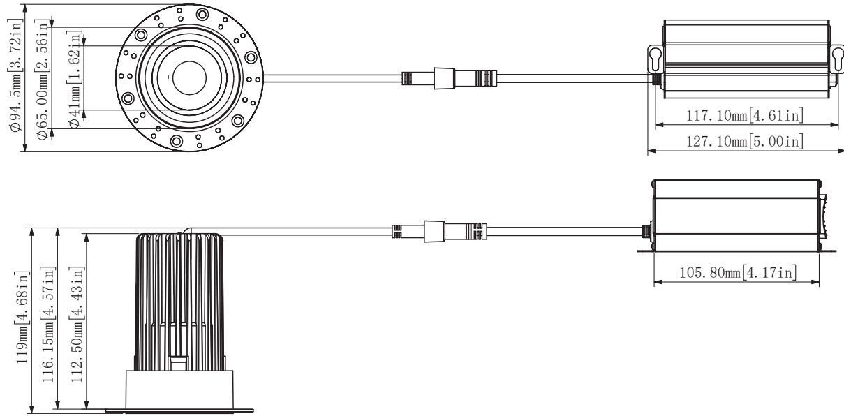
Technical Drawing: 3.72" (D) x 4.68" (W)
