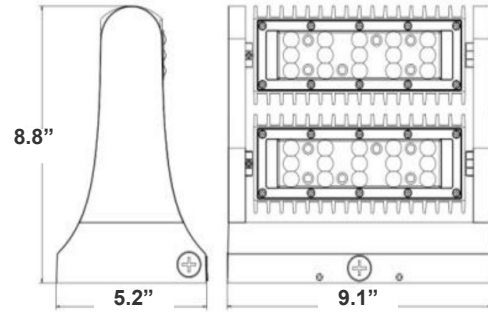
8.8"(H) x 5.2"(W) x 9.1"(L)
