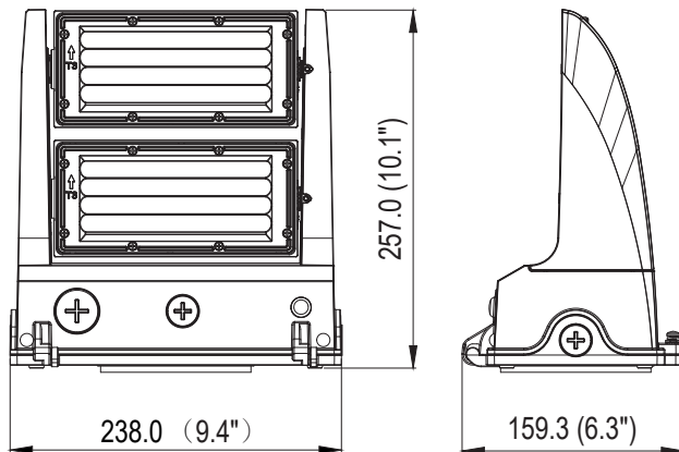
Technical Drawing: 6.3" (D) x 9.4" (W) x 10.1" (H)
