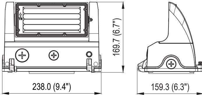
Technical Drawing: 6.3" (D) x 9.4" (W) x 6.7" (H)
