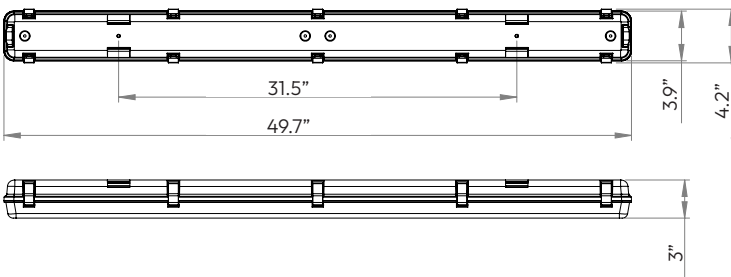
Technical Drawing: 3" (D) x 49.6" (W) x 4.2" (H)
