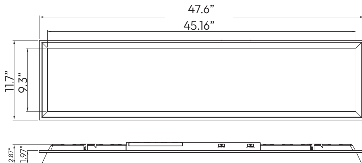
Technical Drawing: 2.87" (D) x 47.6" (W) x 11.7" (H)
