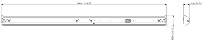
Technical Drawing: 3.6" (D) x 92.8" (W) x 6.2" (H)
