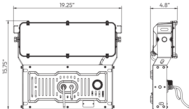
Technical Drawing: 15.75" (H) x 19.25" (W) x 4.8" (D)
