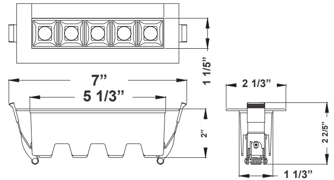
2"(H) X 7"(W) X 1 1/5"(D)
