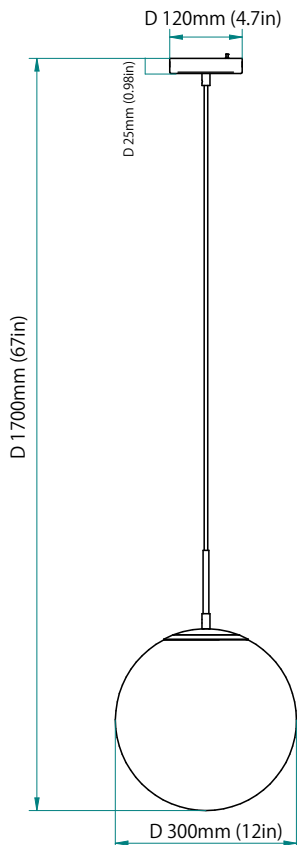
Technical Drawing: 12" (D) x 4.7" (W) x 67" (H)
