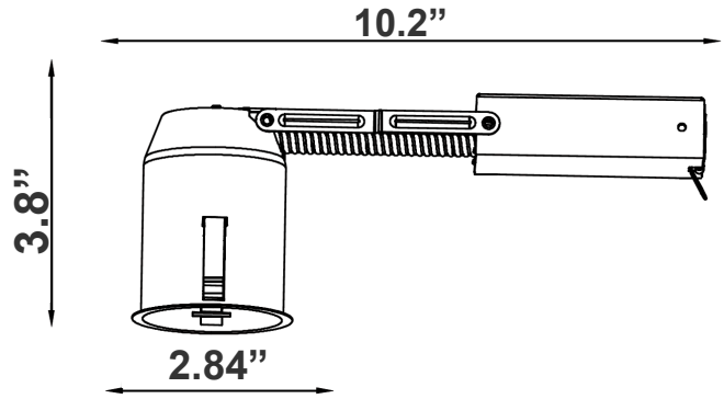
3.8"(H) x 10.2"(W) x 2.84"(D)
