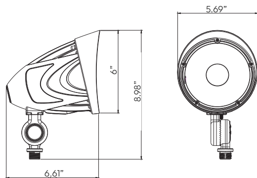
Technical Drawing: 8.98" (H) x 6.61" (W) x 5.69" (D)
