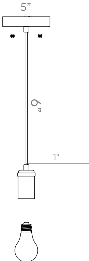
Technical Drawing: 5" (W) x 6" (H) x 1" (D)
