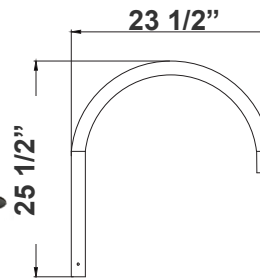
DAB-BA 23 1/2"(W) x 25 1/2"(H)
