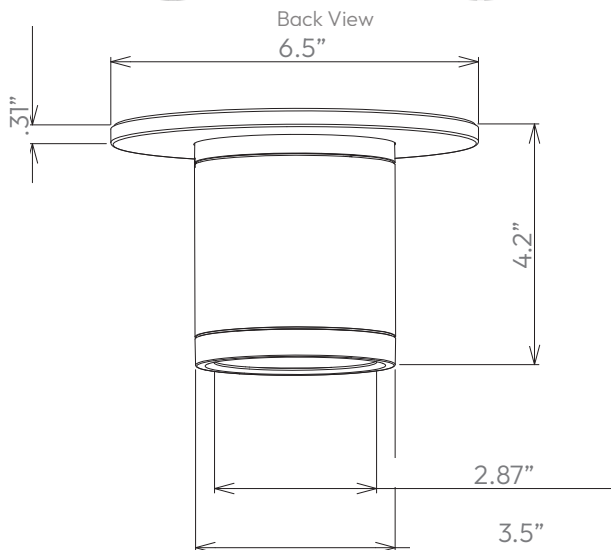
Technical Drawing: 6.5" (D) x 3.5" (W) x 4.2" (H)
