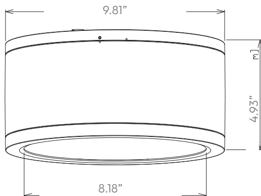
Technical Drawing: 9.81" (D) x 8.18" (W) x 4.93" (H)
