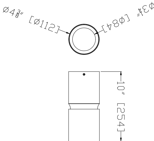
Technical Drawing: 10" (H) x 4-3/8" (D)
