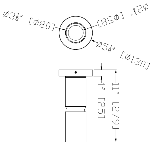
Technical Drawing: 5 -1/8" (W) x 11" (H) x 1" (D)
