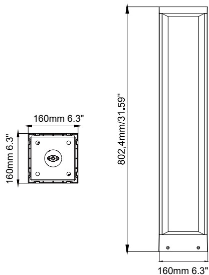
Technical Drawing: 6.3" (D) x 6.3" (W) x 31.59" (H)
