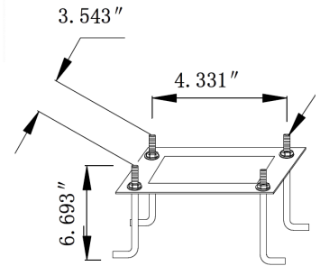
BOL-602-ABK 6.693"(H) X 4.331"(W) X 3.543"(D)
