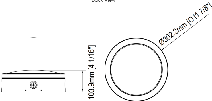
Technical Drawing: 4 1/16" (H) x 11 7/8" (D)
