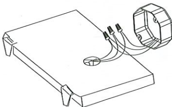
Fig.A (J-Box)
