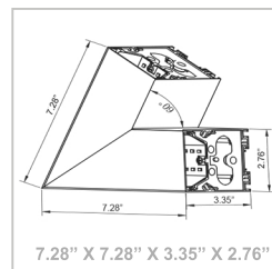
60° Corner Module
