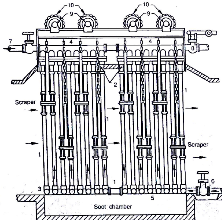
Fig. 3.16 Economiser
