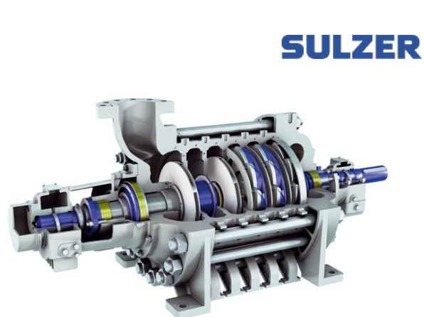
Bomba horizontal multietapas Serie MC
