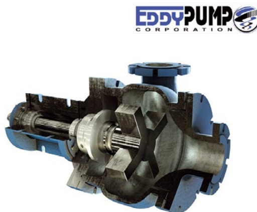
Bomba para lodos
