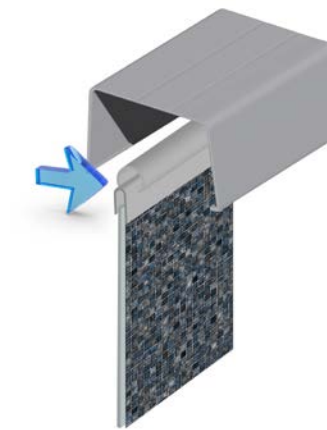
Toiles accrochées U-bead liners
