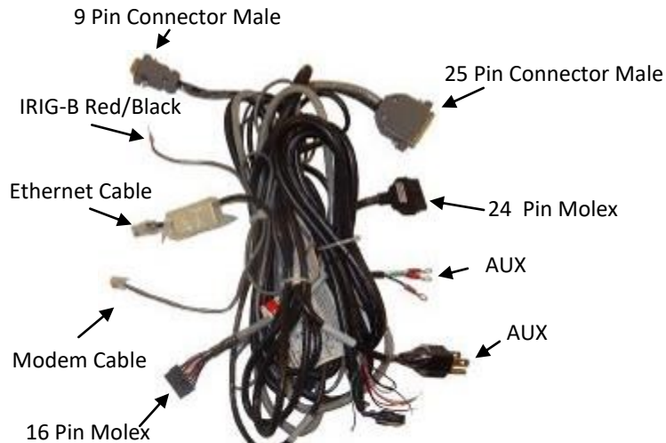
QK1 Cable
