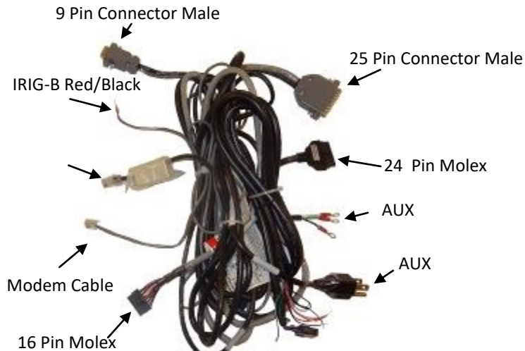
QK1 Cable
