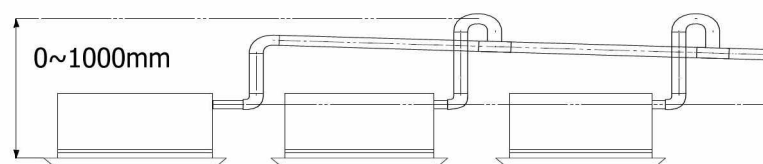
Połączenia typ 2 rur skroplin
