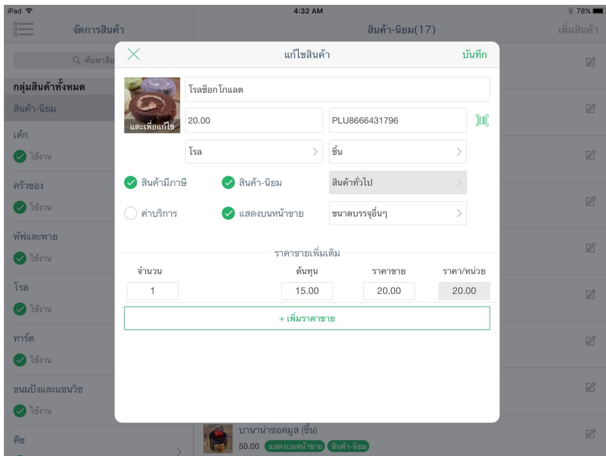
รูปแสดงหน้าการใส่ข้อมูลหลักของสินค้า
