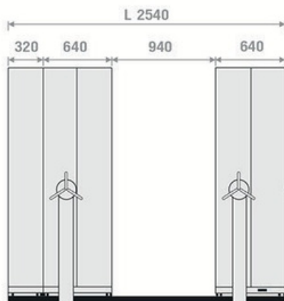
ด้านข้าง CPT-105
