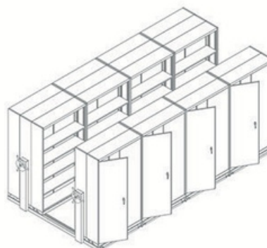
CPT-405 (4 แถว)
