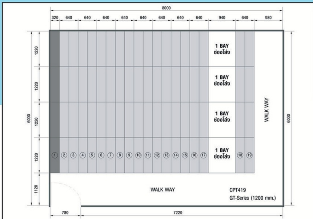
ระบบตู้เอกสารรางเลื่อน (GT Series-120)
