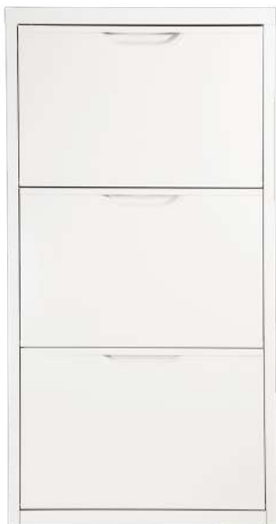
SW-103 : ตู้รองเท้า 3 ลี้นชัก บานสวิง Swing cabinet - 3 doors Size: W60 x D20 x H116.8 cm. 6 adjustable dividers, 3 removable shelves.
