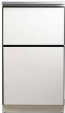
DB-101 : ตู้ครัวท็อปสแตนเลส 1 ลื่นชัก, 1บานเปิด Kitchen cabinet stainless top Size: W50 x D60 x H90 cm. 1 drawer ,1 door , 1 shelf.
