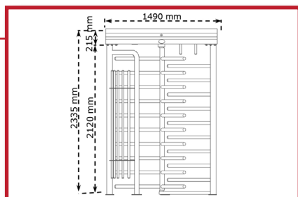
Tegning med mål. Passeringshøyde er 2 m. Passeringsbredde 0,6 m.
