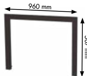
Cadre à 3 côtés de 5 cm. pour BR90D-S. Ref.: M3-BR90D
