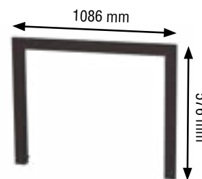
Cadre à 3 côtés de 5 cm. pour BR100-S. Ref.: M3-BR100
