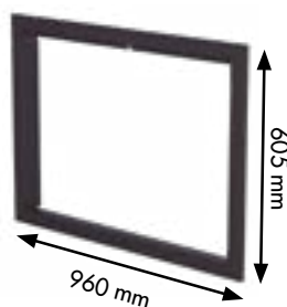
Cadre à 4 côtés de 5 cm. pour BR90D-S. Ref.: M4-BR90D
