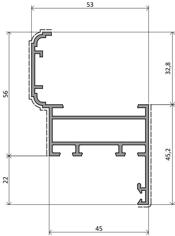
NX10285 | 0,920 Kg/m
