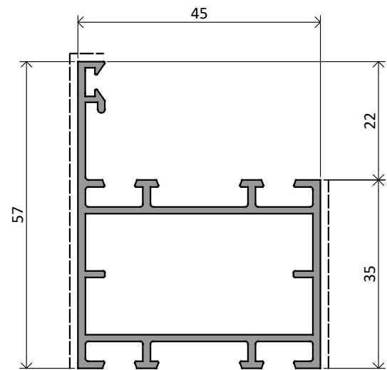
NX2769 | 0,886 Kg/m
