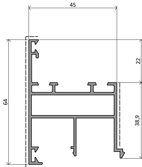
NX420 | 0,931 Kg/m
