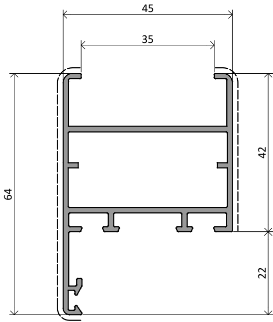
NX3546 | 0,893 Kg/m
