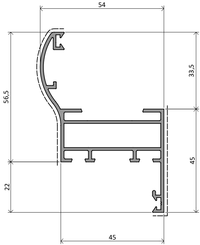
NX10471 | 0,910 Kg/m
