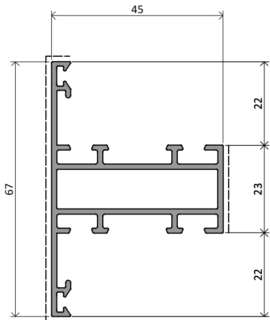
NX32 | 0,911 Kg/m
