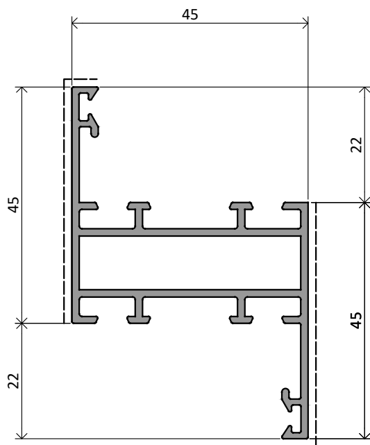
NX33 | 0,911 Kg/m
