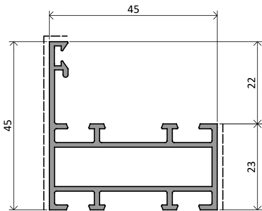
NX36 | 0,737 Kg/m
