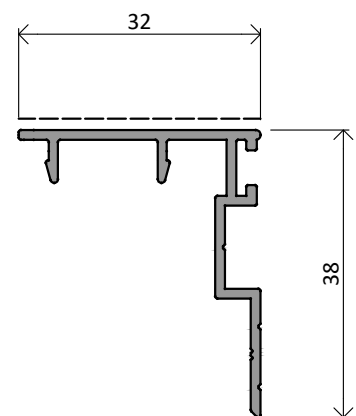
NX10593 | 0,319 Kg/m
