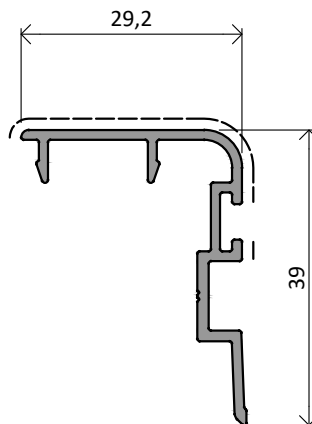
NX10467 | 0,321 Kg/m
