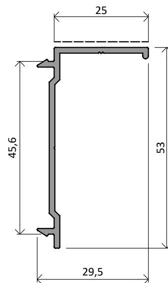
NX10592 | 0,354 Kg/m
