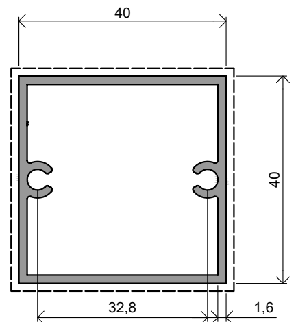
NX10489 | 0,748 Kg/m
