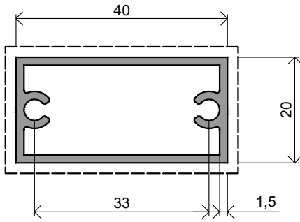
NX10333 | 0,546 Kg/m
