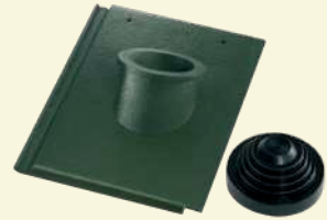
ชุดกระเบื้องปล่อง เอสซีจี รุ่น เวิร์สทีจ
