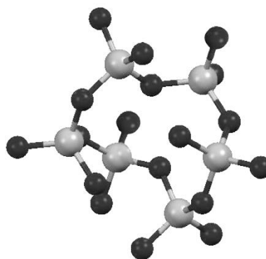
Struktura \beta -GeO 2
