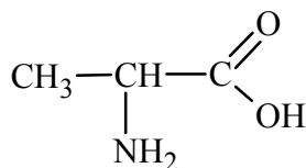
alanina (Ala)
